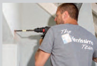
1 / Percer les trous et adapter la fixation des tiges filetées en fonction du support
