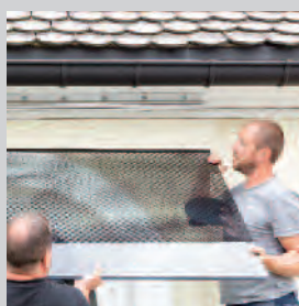
2 / Enfiler le profilé de protection des arêtes sur le verre (respecter le sens) et insérer ensuite la vitre dans le profilé de la marquise en plaçant les trous de perçage en bas.
