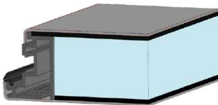
Coupe de SOLOBLOC 68.1 avec complexe isolant stabilisé
