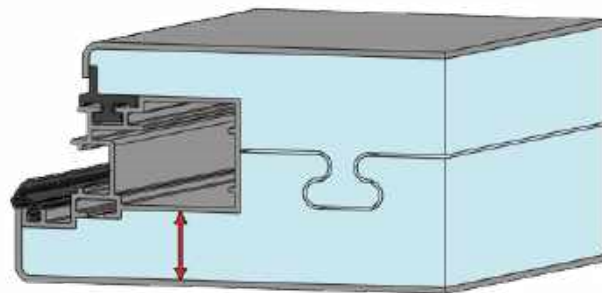
Coupe de SOLOBLOC 80.2, brevet Oméga et des différentes adaptations aux dormants
